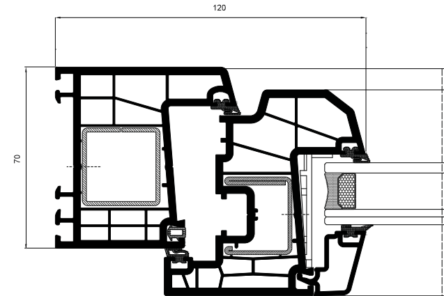
SECCIÓN SEMIENRASADA
