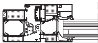
Schüco Fenster AWS 60 FR 30 Horizontalschnitt, Maßstab 1:4 Schüco Window AWS 60 FR 30 Horizontal section detail, scale 1:4
